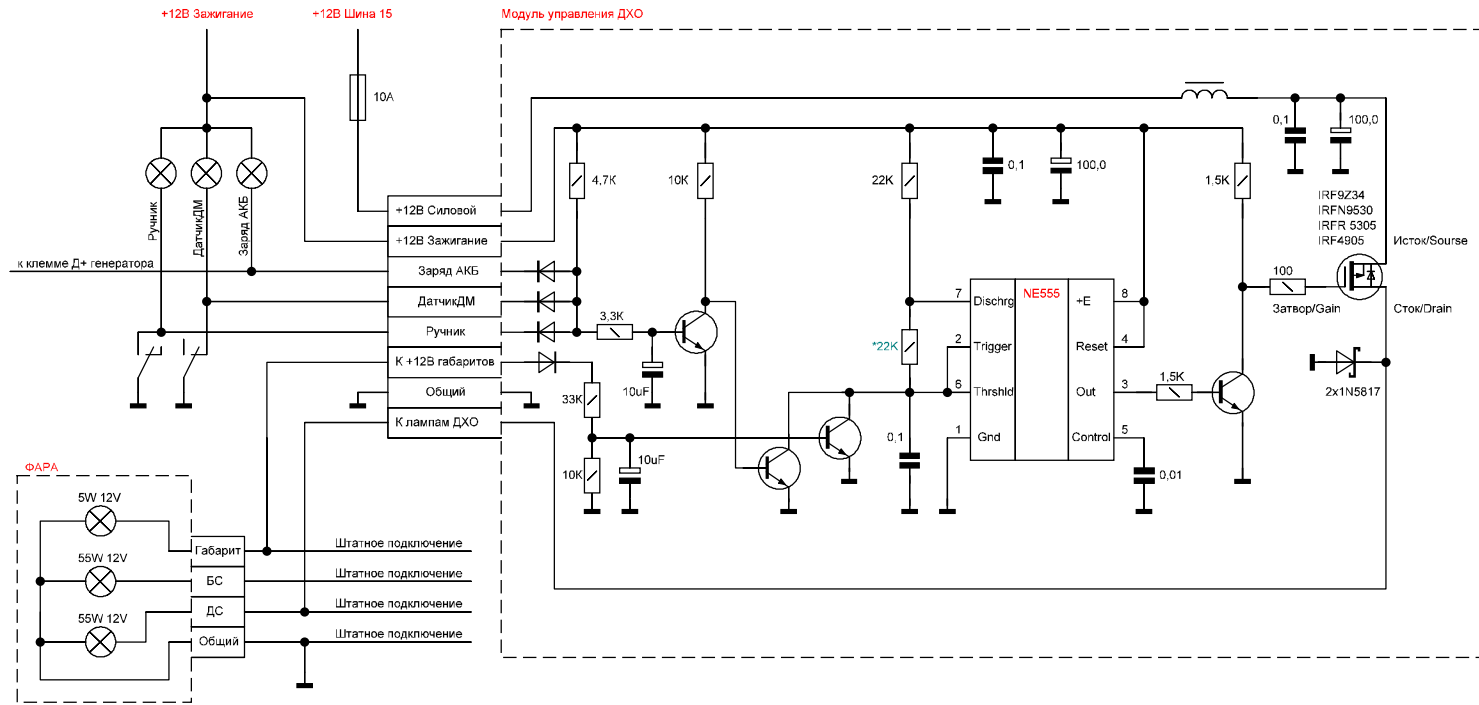
Вариант использования N-проводимости полевика
