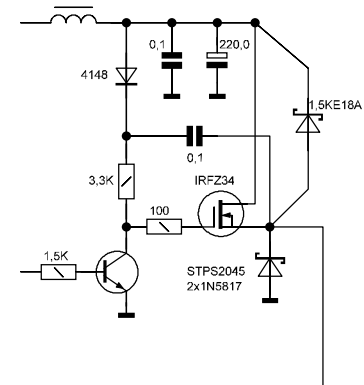
Вариант использования N-проводимости полевика
